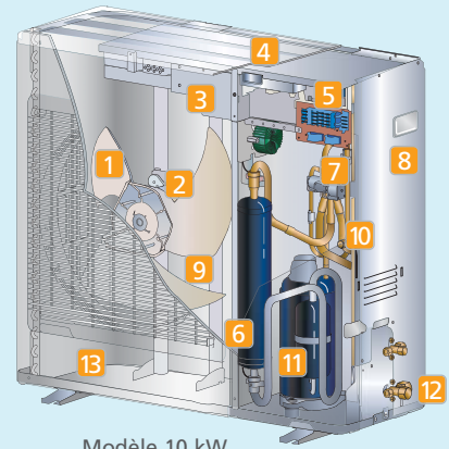
Modèle 10 kW
